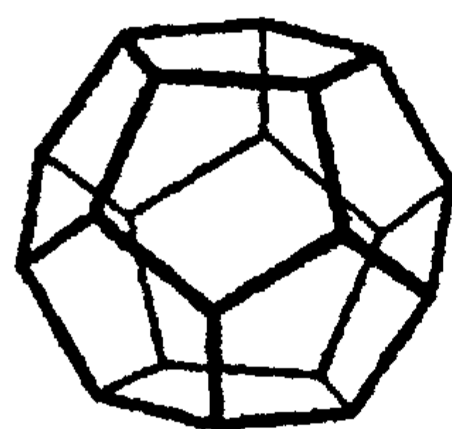
ذو الاثنى عشر سطحاً
