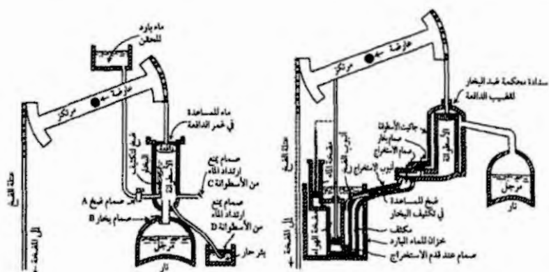
مخطط للآليات الأساسية في محرك نيوكومن الجوي (إلى اليسار) والمكثف المستقل لـ واط (إلى اليمين)
