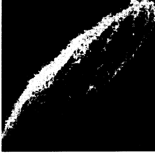
شكل ٣-١٦: حيوان البراميسيوم: لاحظ الأهداب الشبه شعرية التي تُستخدم في السباحة، وهذه الأهداب تشكل الأطراف الخارجية لهيكل خلية البراميسيوم.
